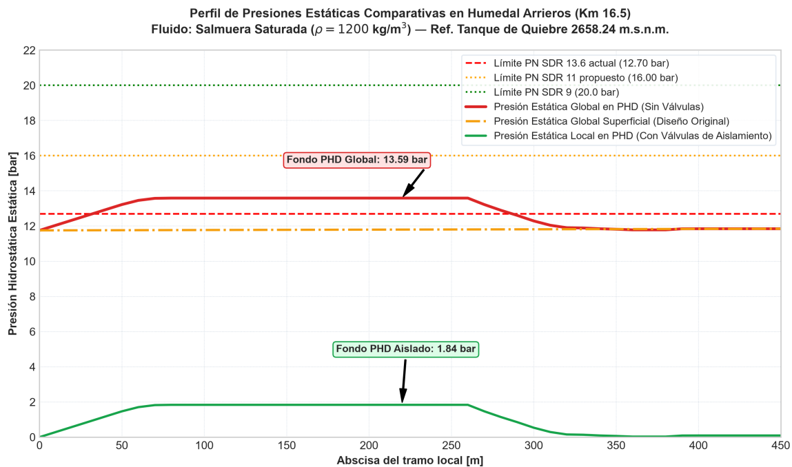
Figura 2: Perfil de presiones estáticas hidrostáticas comparativas en el tramo Km 16.5 (Humedal Arrieros) para el escenario global y local aislado en salmuera saturada.
